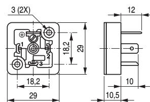
Base de Sobrepor tipo F (para conector quadrado)
