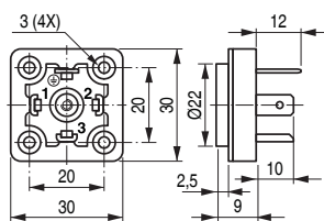
Base de Embutir tipo C (para conector quadrado)
