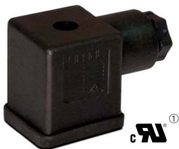
Conector Quadrado DIN 43650 forma A
