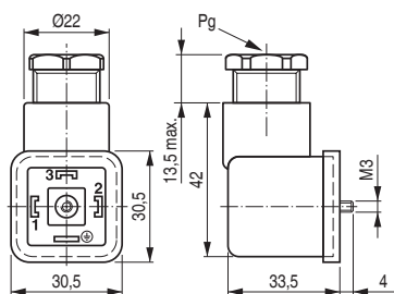
Conector Quadrado DIN 43650 forma A
